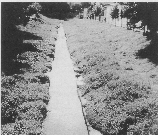
Mistelbach przed renaturalizacją w formie prostoliniowej rynny [1].
