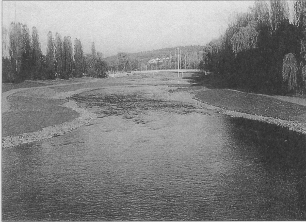
Enz po renaturalizacji. Zburzona powierzchnia wody wskazuje na bardziej zróżnicowane zachowanie prądu niż w stanie wyjściowym. Rzeka staje się lepiej natleniona. Fot. Bernhart [2].
