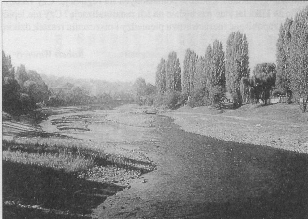
Na rozszerzeniach koryta zostały wykonane wyspy i zawężenia koryta. Obydwa te elementy nadają różną dynamikę płynącej wodzie i ofiarowują bardziej bogate siedliska. Fot. Mayer-Peters [2].
